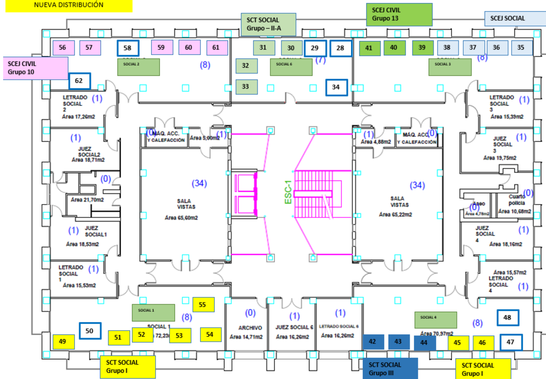
Planta 1ª
